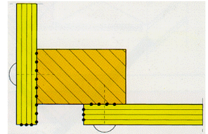
Figuur 10 Goed uitgevoerde hoekaansluiting.
